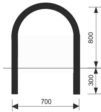
Form Rundbogen
